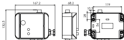
Steuereinheit
